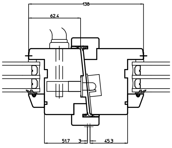
Horizontalsnitt mötesbåge
